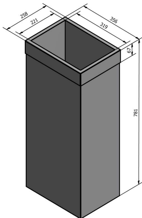
Femund 65 L: art.nr 32028 med std topp 32120
